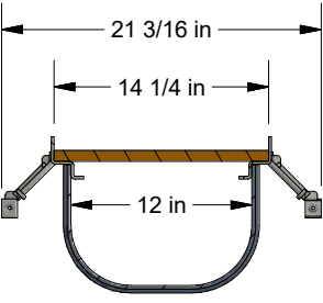
SECTION A-A SCALE 1:14
